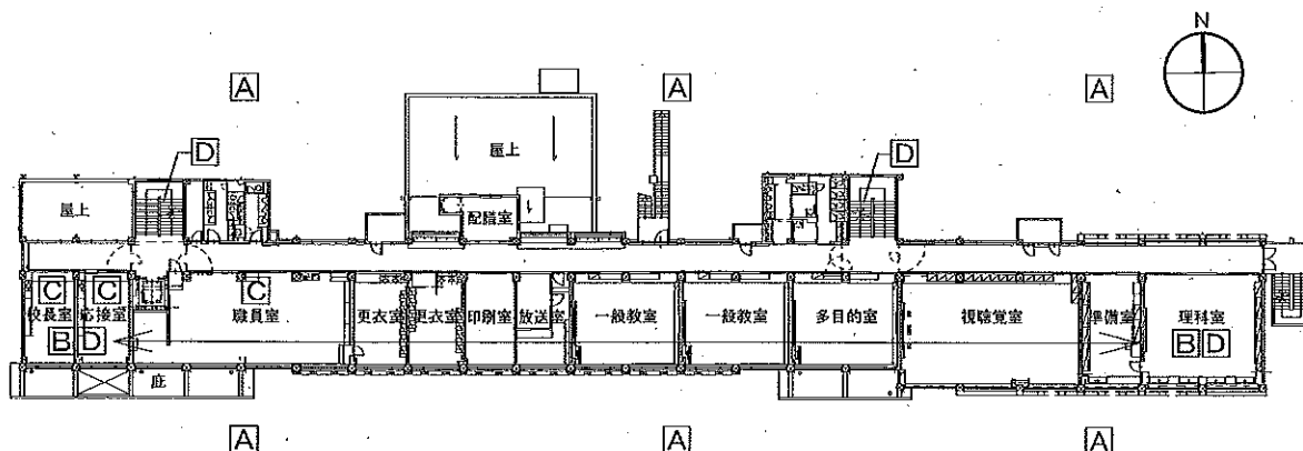
校舎棟 2階平面図
