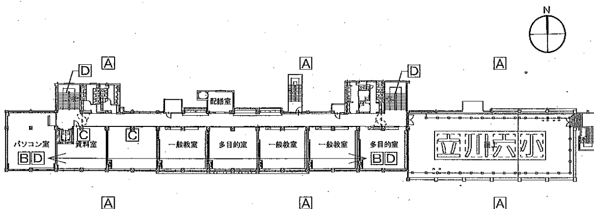
校舎棟 4 階平面図
