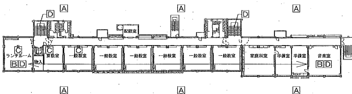
校舎棟 3 階平面図
