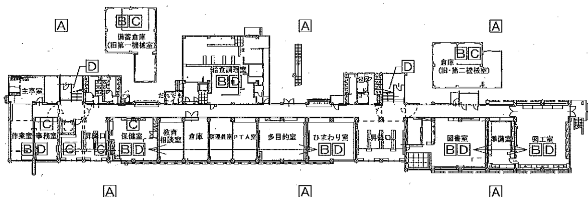
校舎棟 1階平面図
