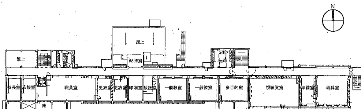
校舎棟2階平面図
