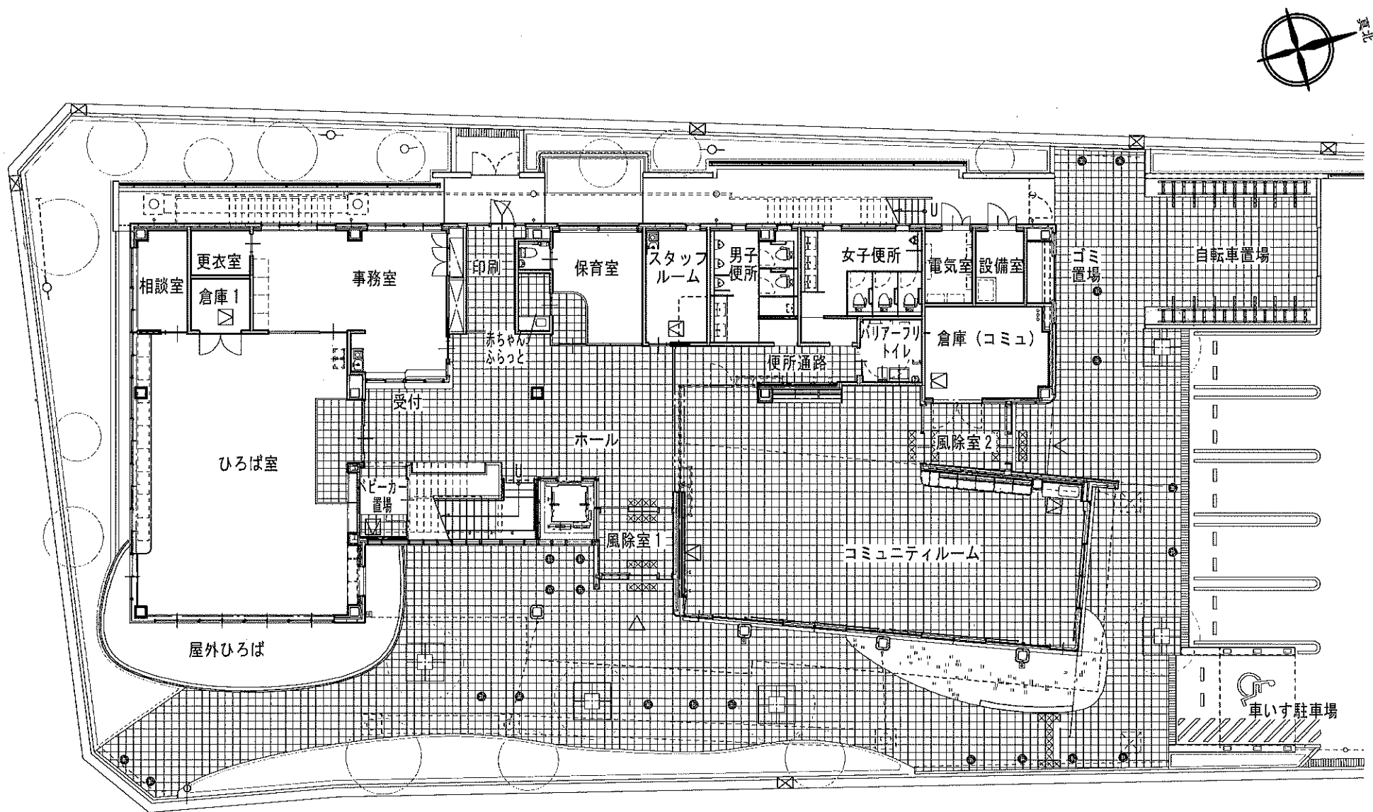
1 階平面図
