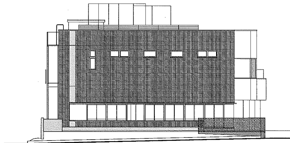
南側立面図
