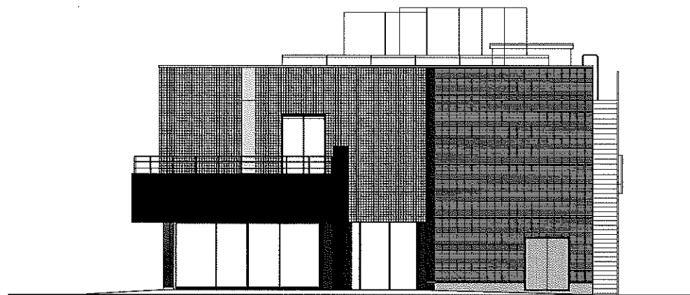
北側立面図
