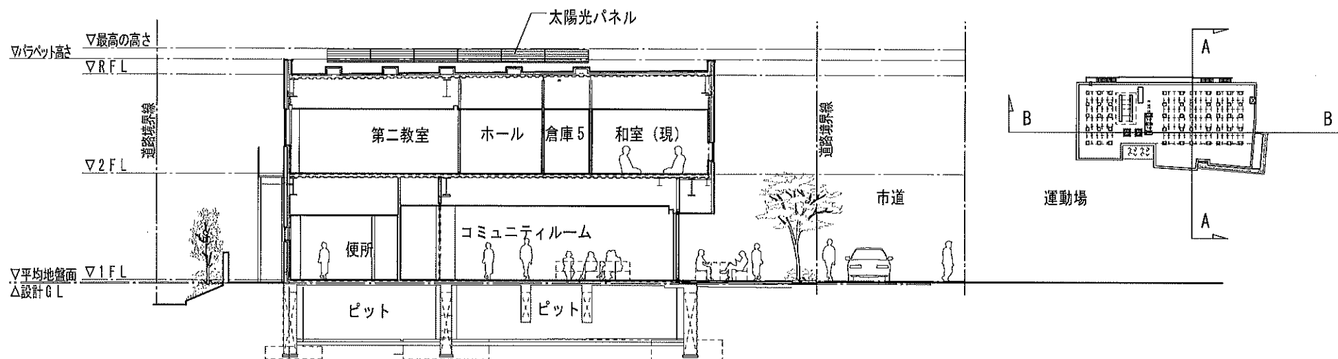
A-A断面図
