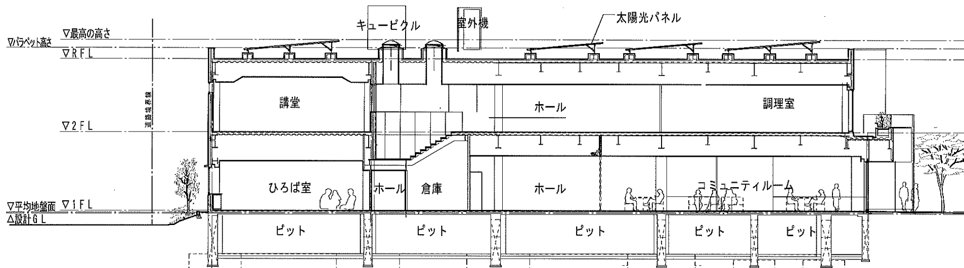
B-B断面図
