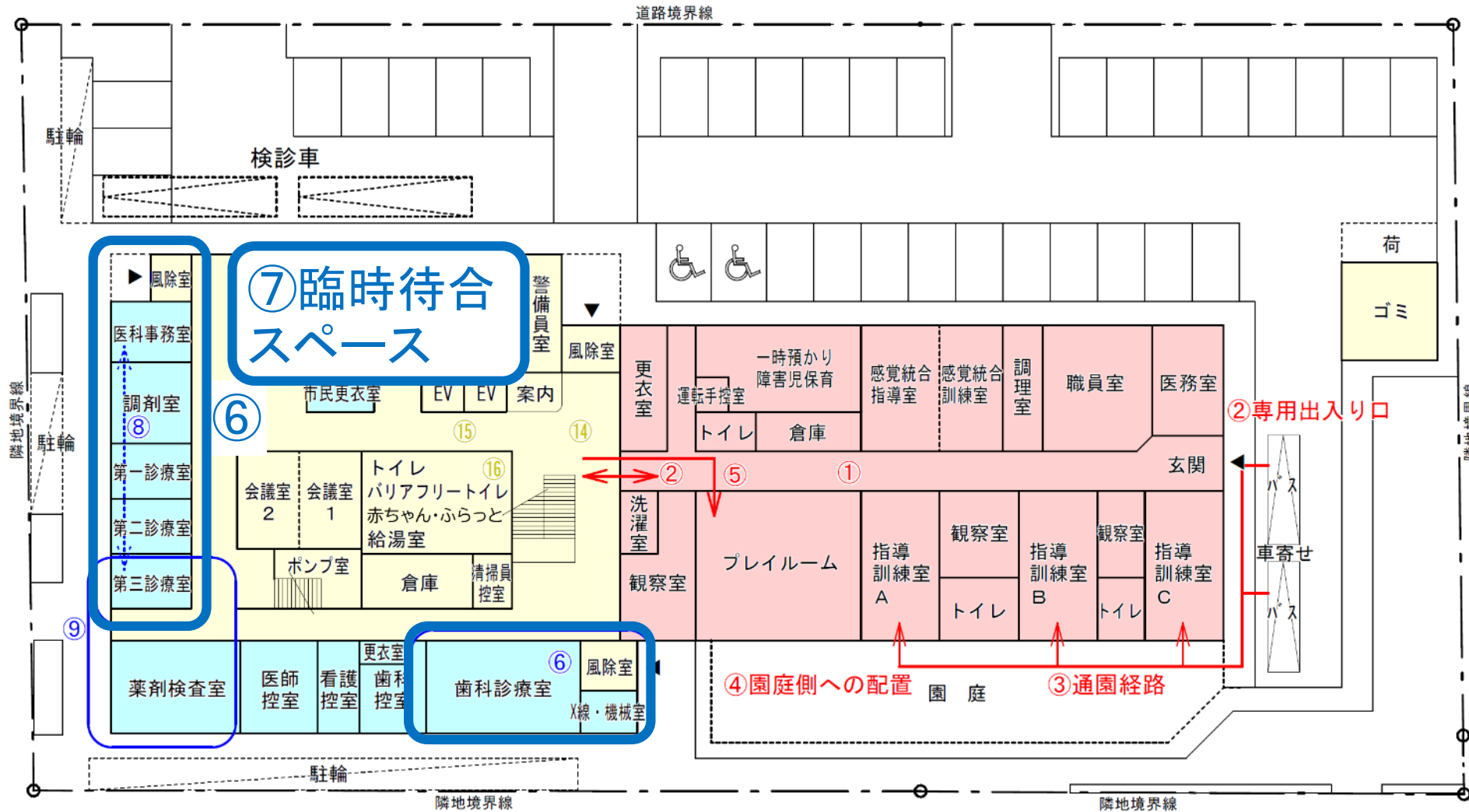
1 階平面図
