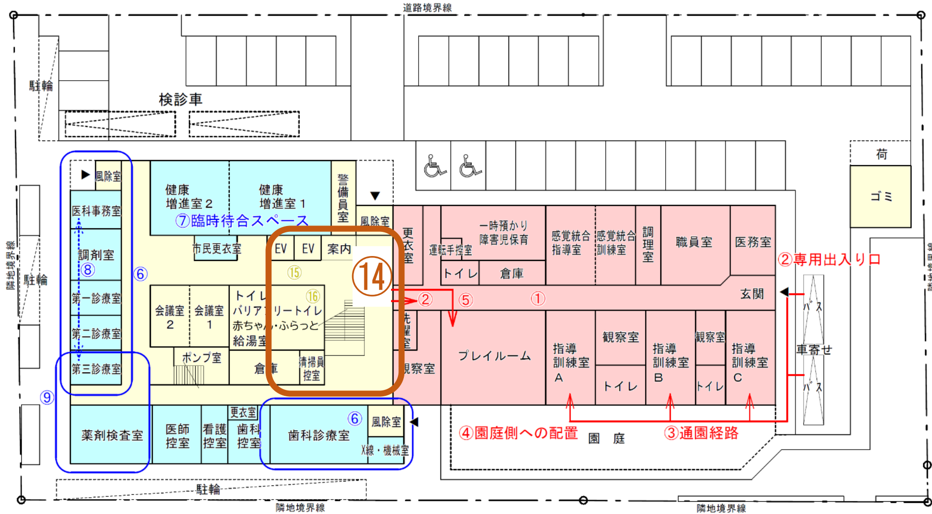
1 階平面図
