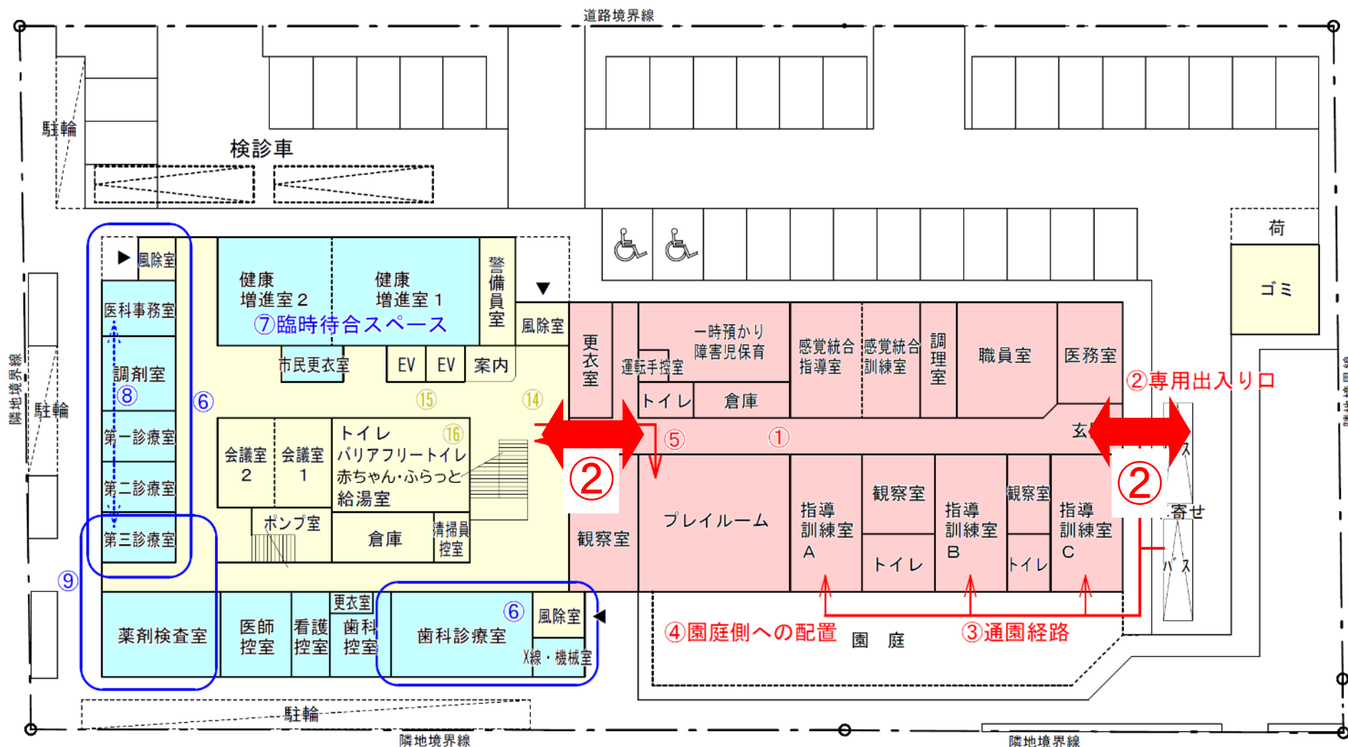
1 階平面図
