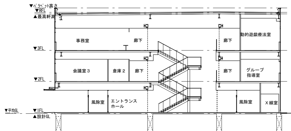
断面図②（南-北）
