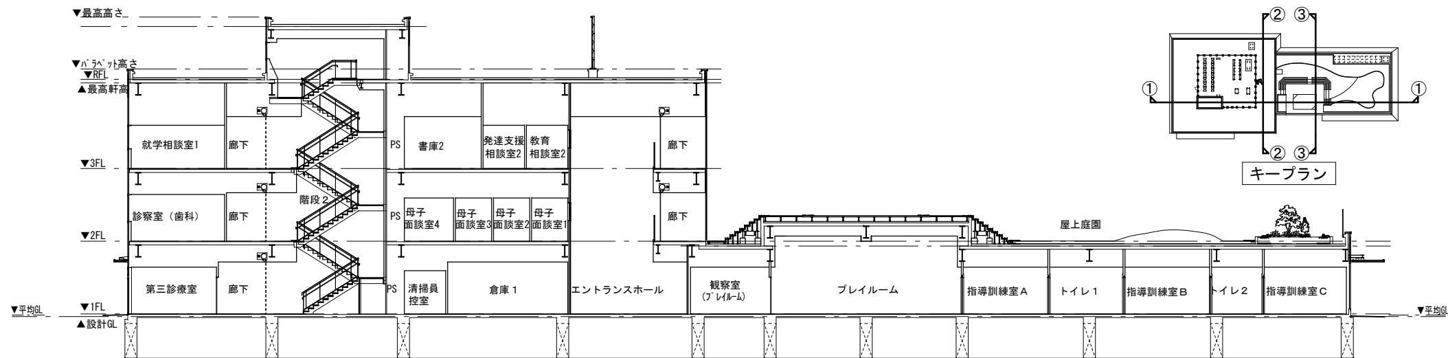
断面図①（東-西）
