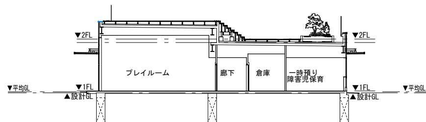
断面図③（南-北）
