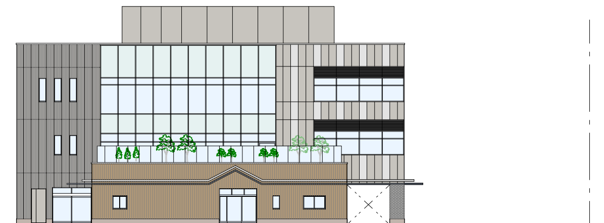
東側立面図
