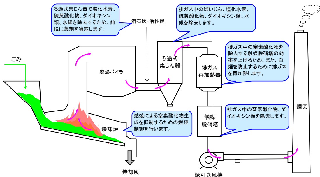
図 7-4 排ガス処理システムのイメージ
