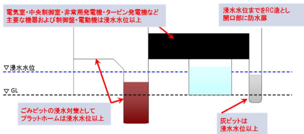
図 10-1 浸水対策
