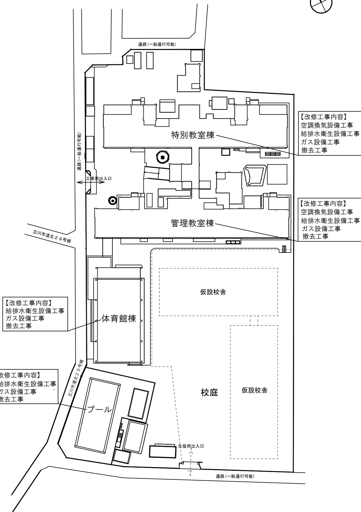
配置図
