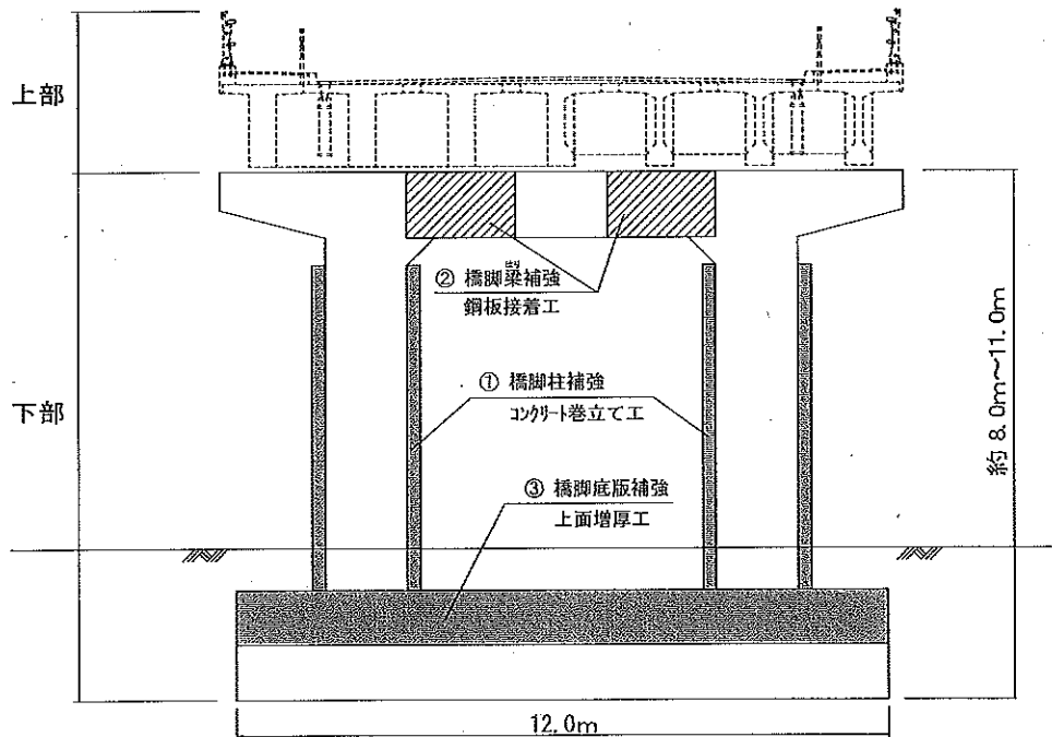
下部工事正面図(P1、P2、P3、P4)
