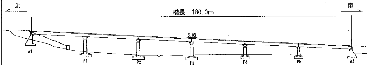
側面図
