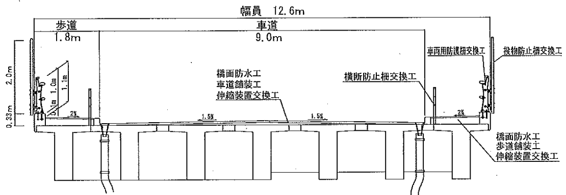
上部工事標準断面図
