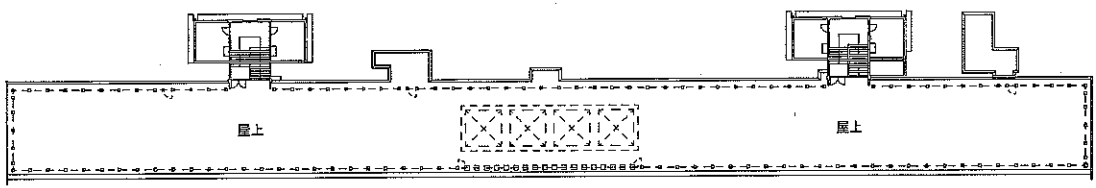
校舎棟R階平面図
