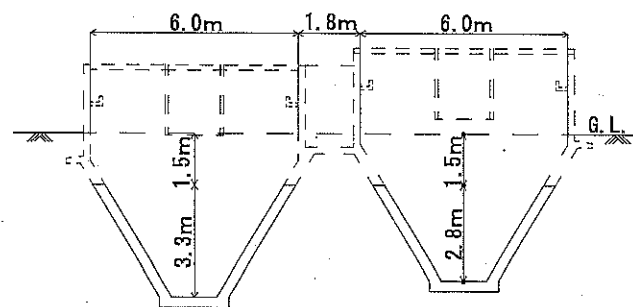
污泥洗净槽断面图
