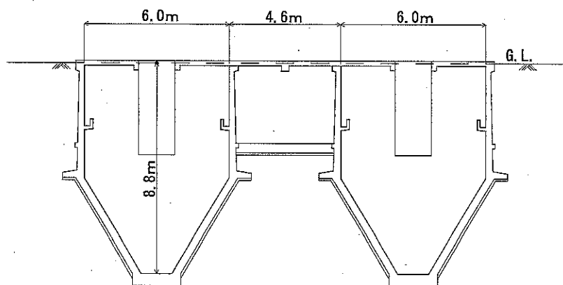
污泥浓缩槽断面图
