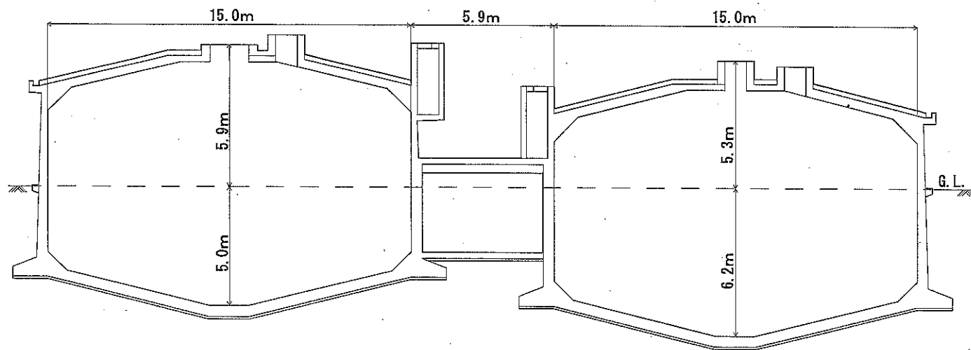
污泥消化槽断面图
