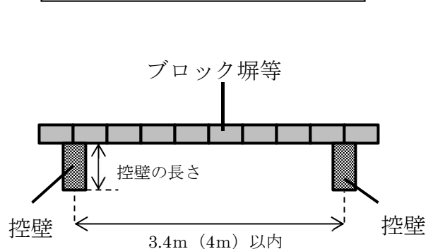
ブロック塀等を上から見た図
