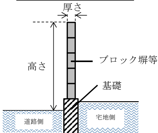
ブロック塀等の断面図
