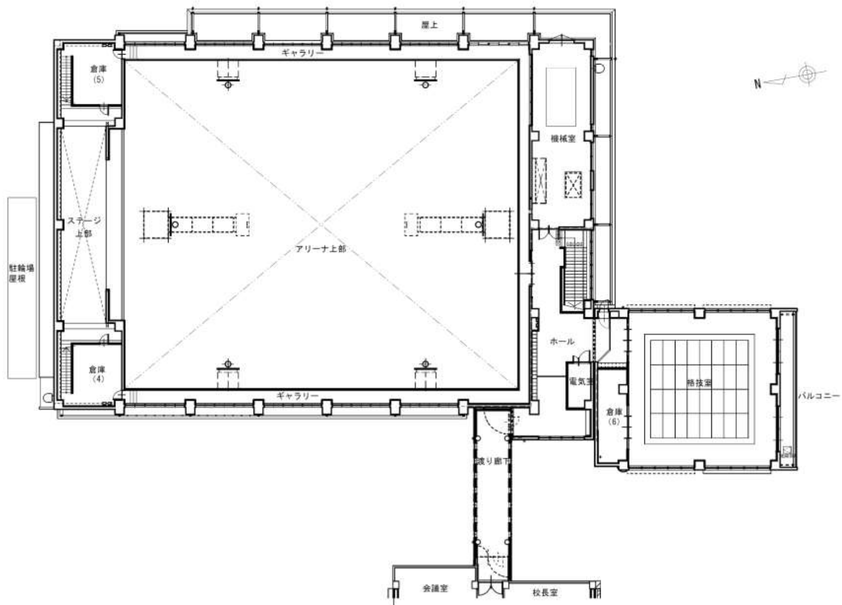
【平面図（2階）】
