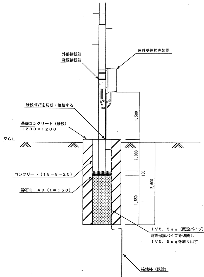
詳細図 (S=1/50)
