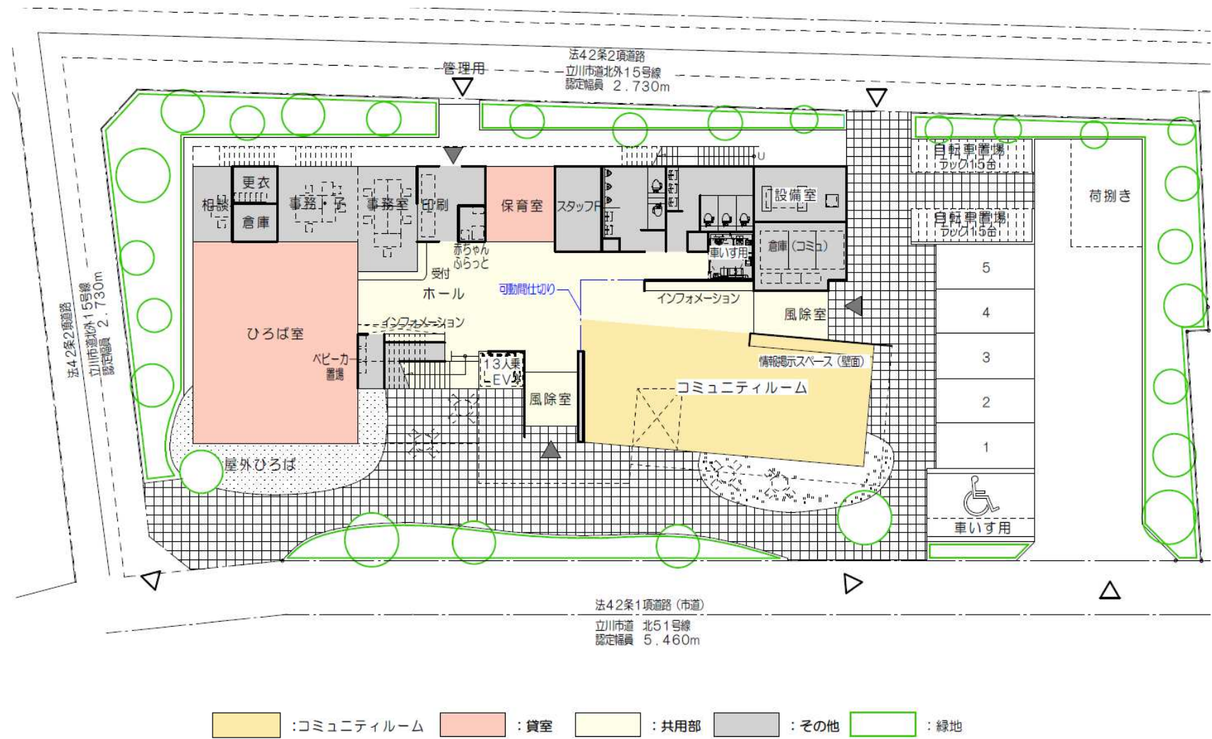
1 階平面図
