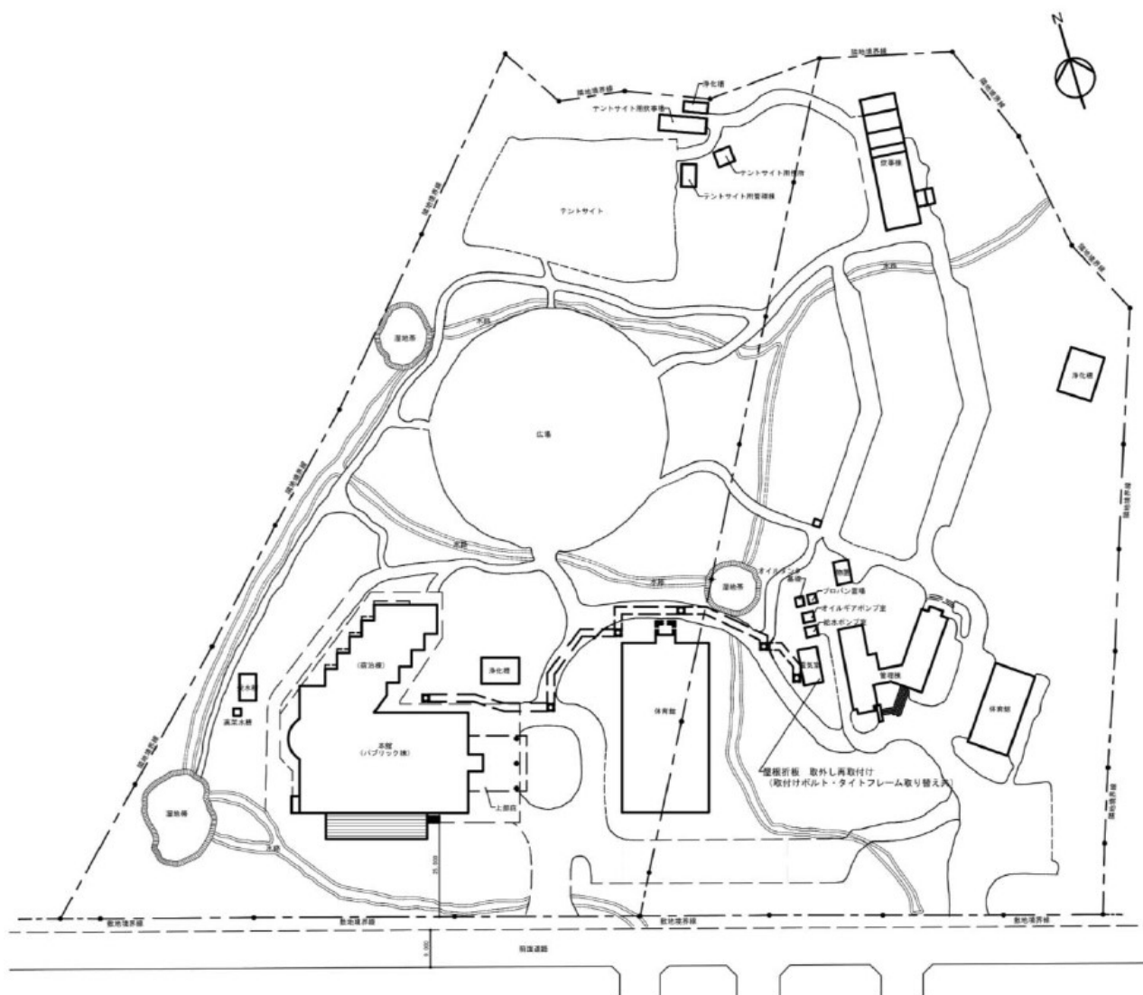
配置図 S=1/500 (A1) 1/1000 (A3)
