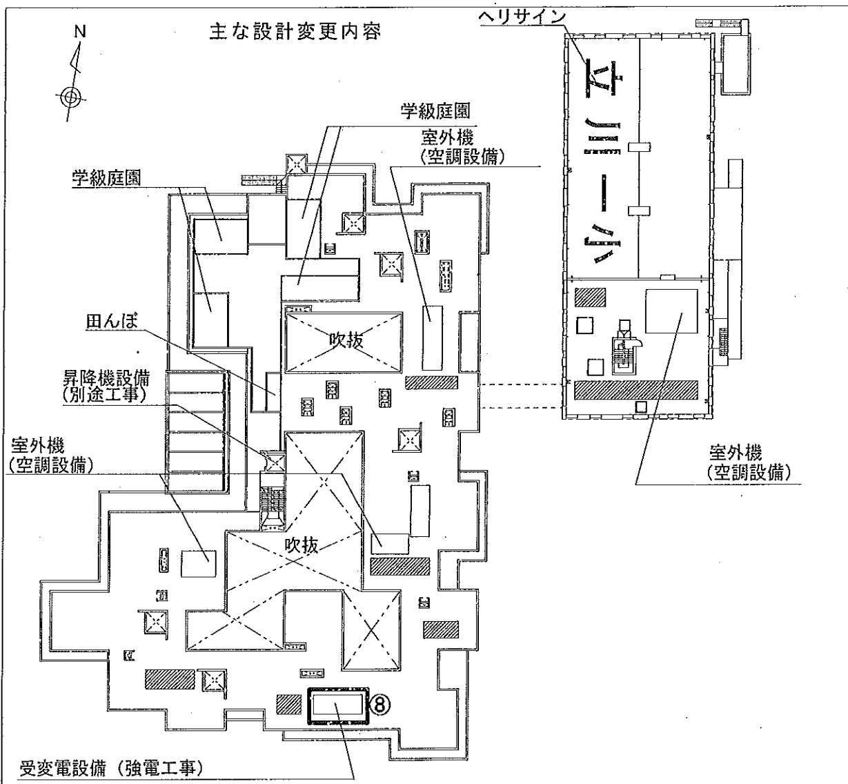
R階平面図 S=1/450
