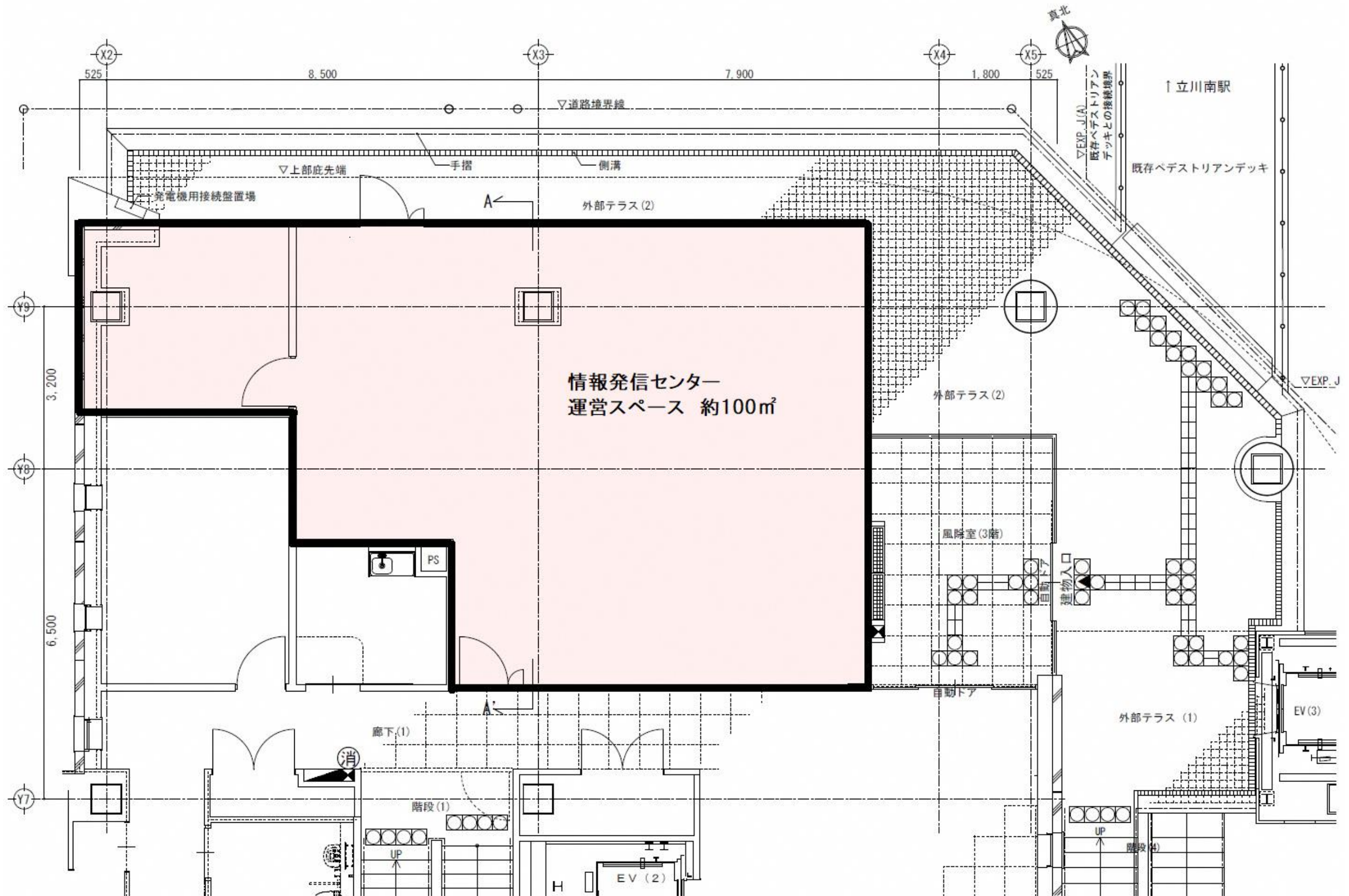
平面図 S=1/100
