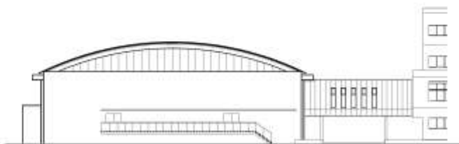
北侧立面图
