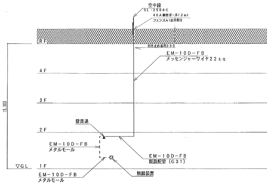
立面図 (S=1/200)
