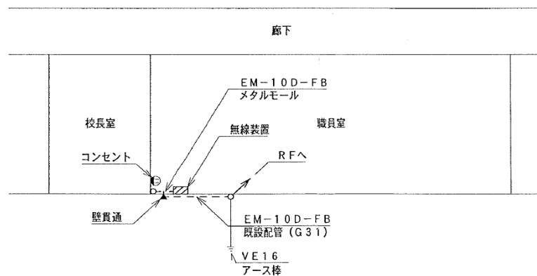
1階平面図 (S=1/200)
