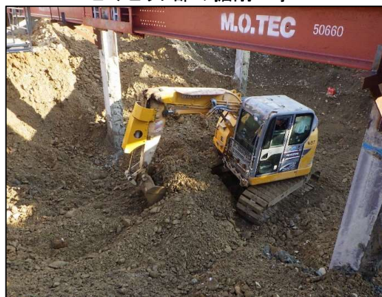
ゴミピット部の掘削工事
